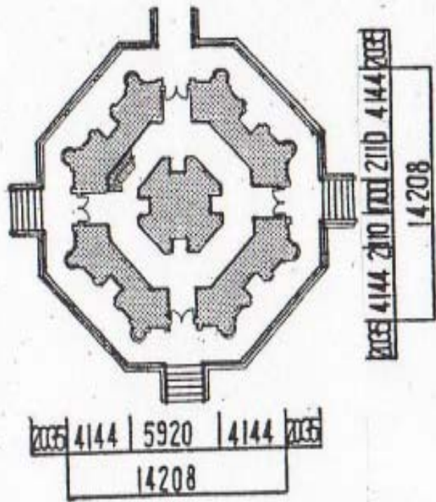
図4 開元寺東塔の平面図
