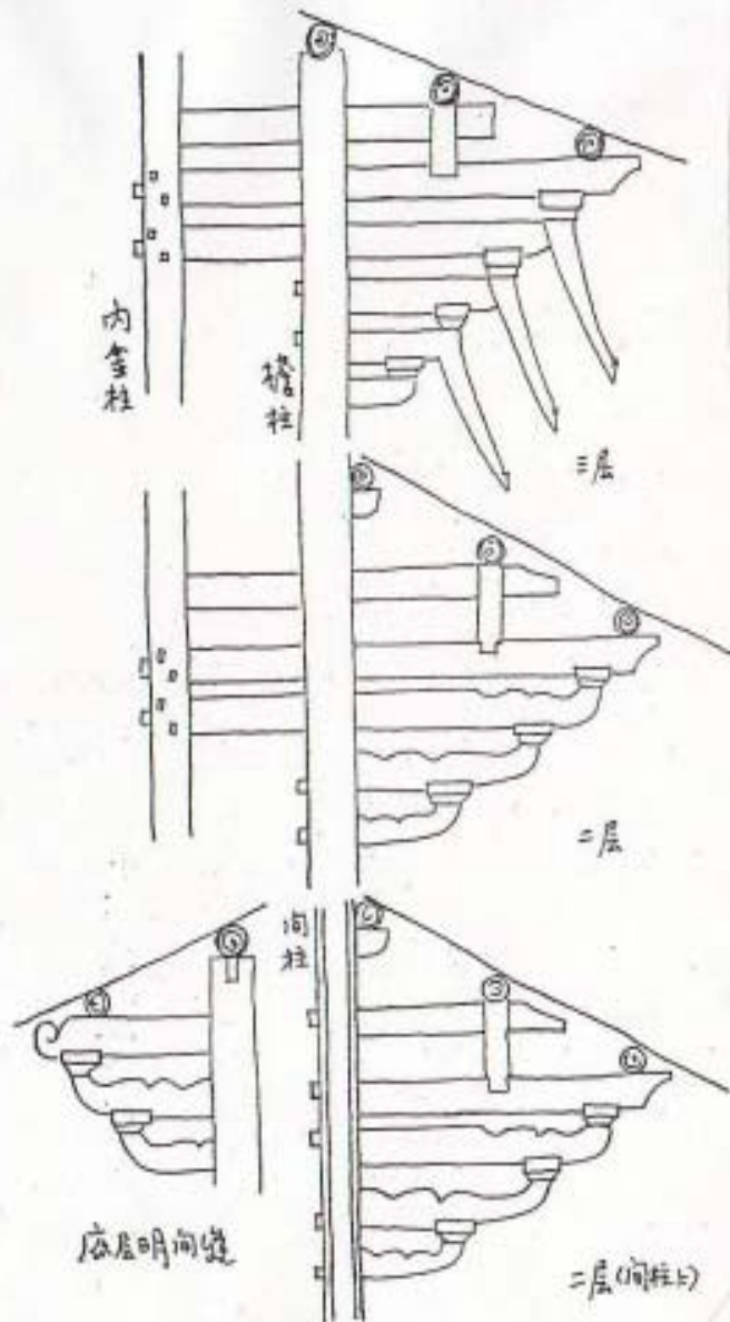
真武閣・一・二・三層の斗組
