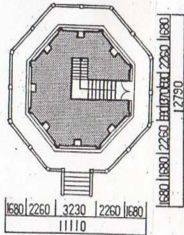
図3 崇妙保聖堅牢塔の平面図
